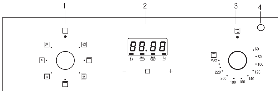
Рис. 1. Панель управления
